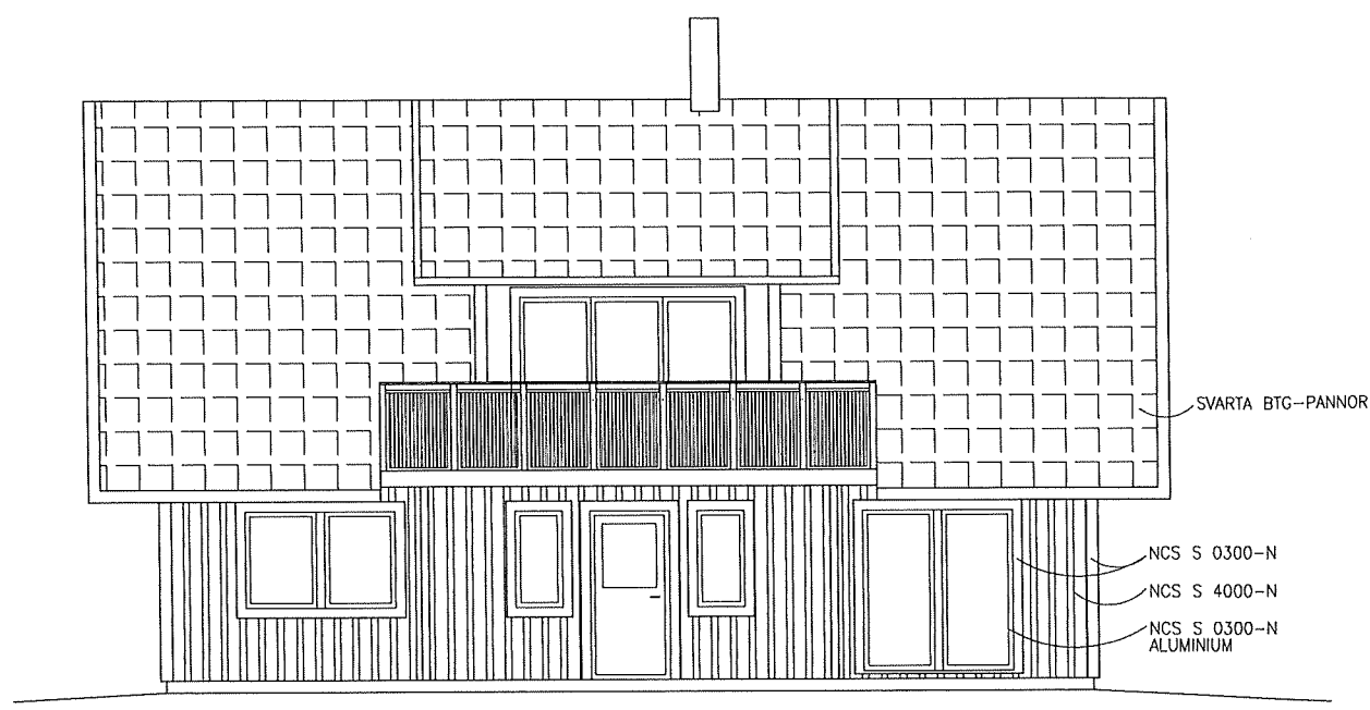
FASAD NORDVÄST
