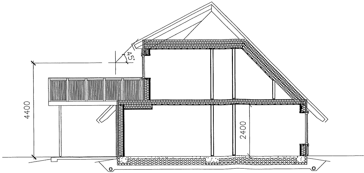
SEKTION A-A
